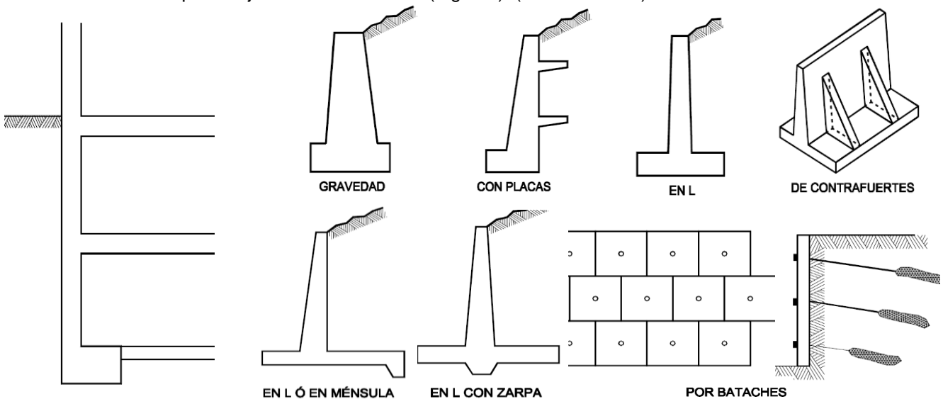
Figura 3.1 Muros de sótano
