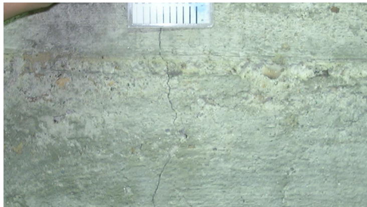
Figura 6. Fisuración por retracción en alzado de muro
